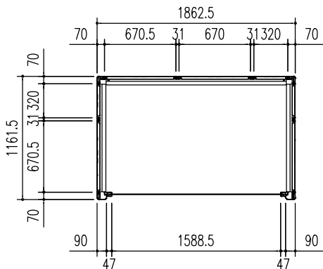
平面図 (S = 1/50)
