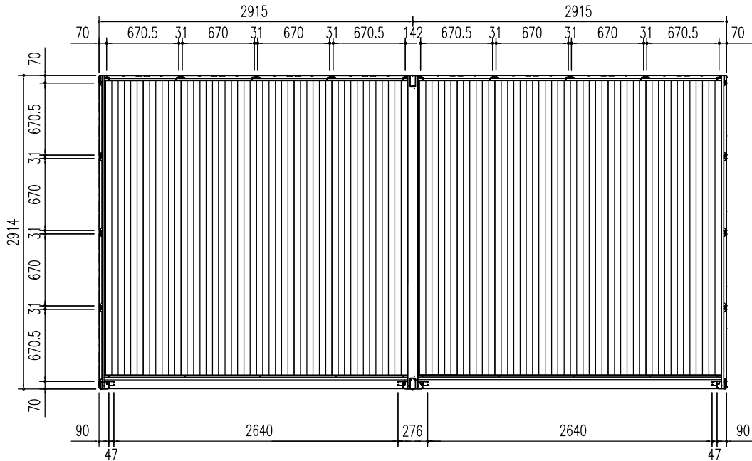
平面図 (S=1/50)
