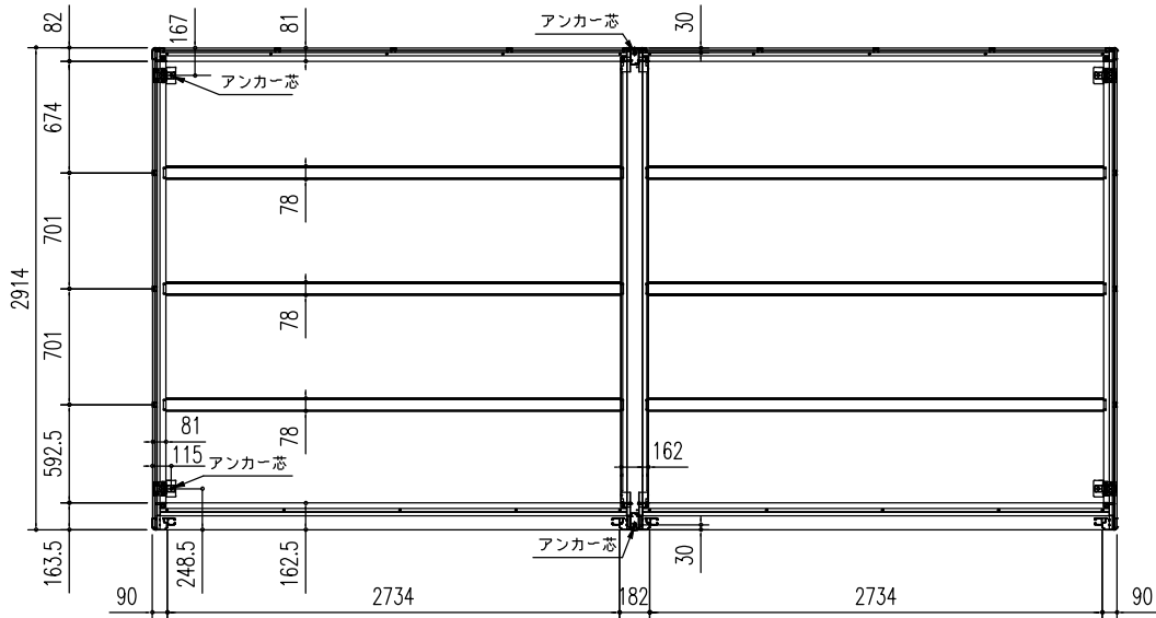
床伏図 (S=1/50)
