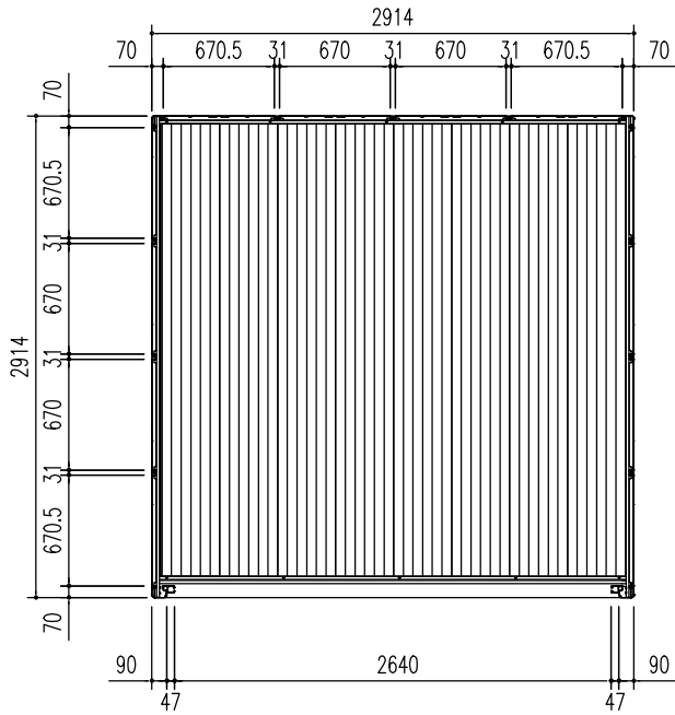
平面図 (S = 1/50)
