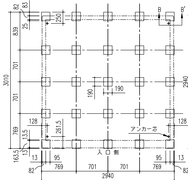
ブロック基礎伏図 (S = 1/50)
