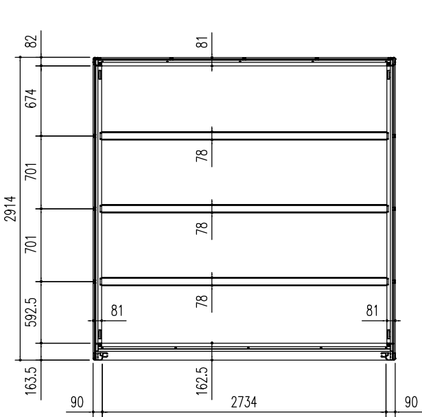
床伏図 (S = 1/50)
