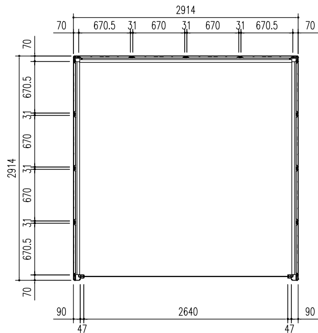
平面図 (S=1/50)
