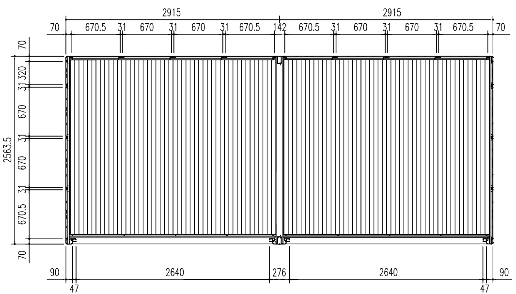
平面図 (S = 1/50)
