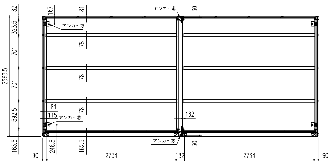
床伏図 (S = 1/50)
