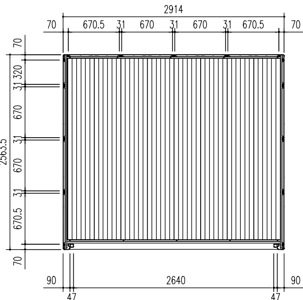
平面図 (S=1/50)
