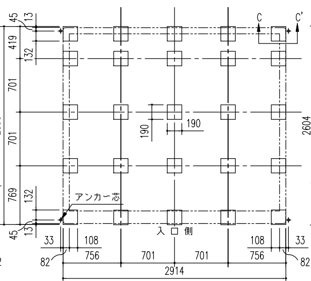
ブロック基礎伏図 (S=1/50)
