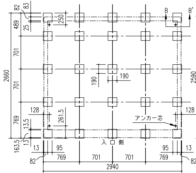
ブロック基礎伏図 (S=1/50)
