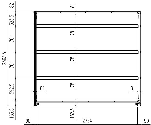
床伏図 (S=1/50)
