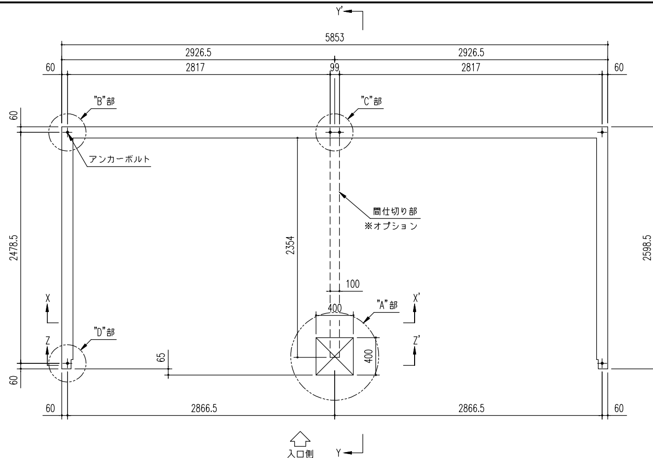
基礎伏図 (S=1/40)
