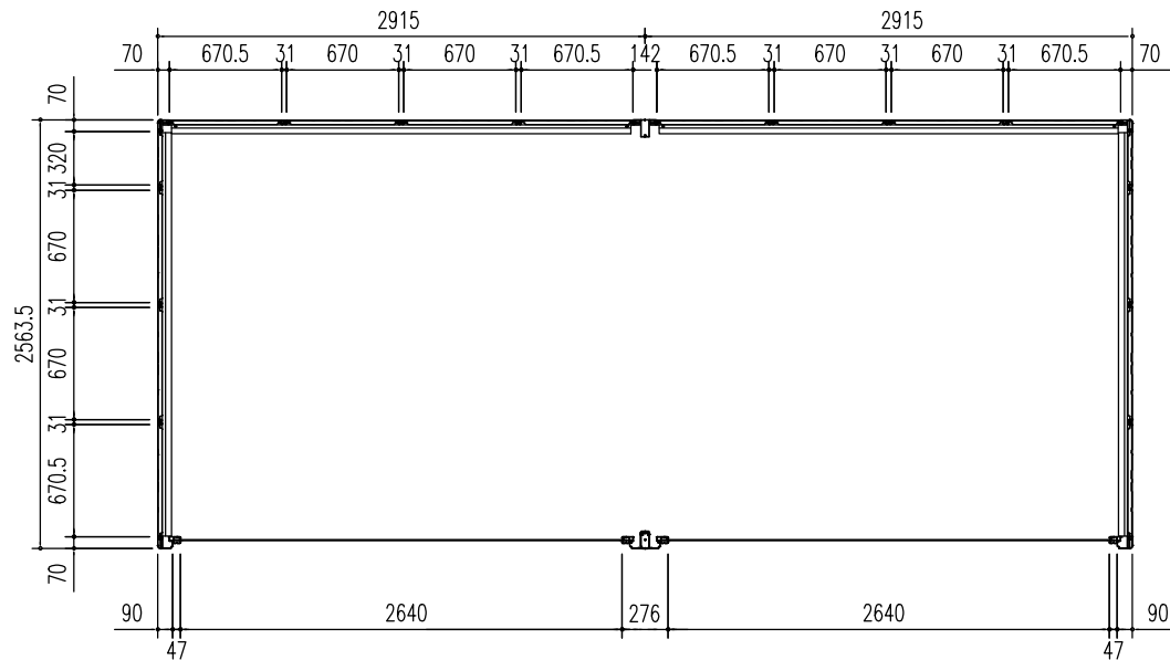
平面図 (S = 1/50)
