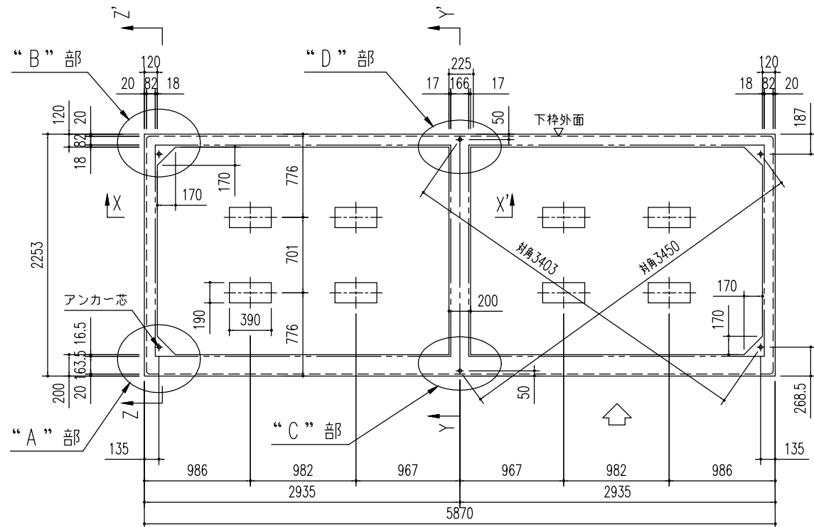
基礎伏図 (S=1/50)
