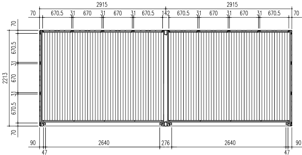
平面図 (S = 1/50)
