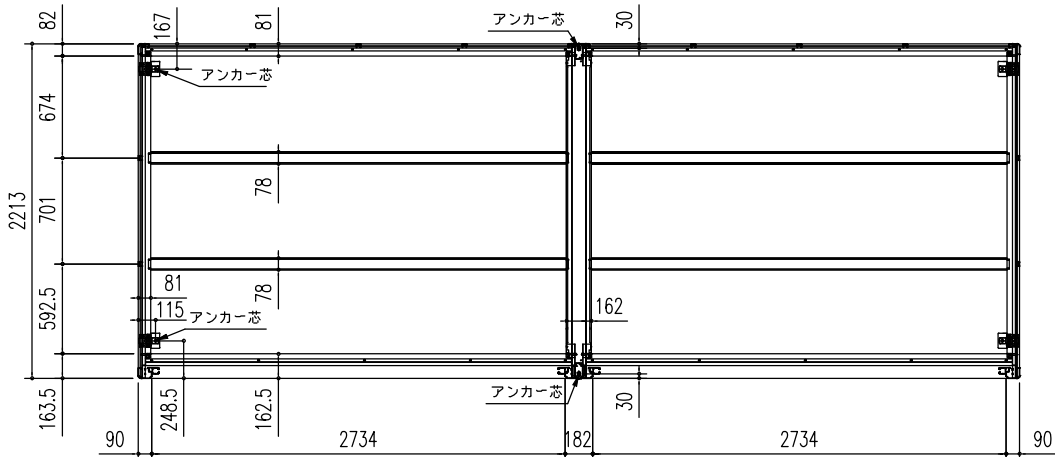
床伏図 (S = 1/50)
