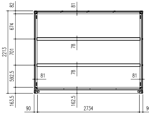
床伏図 (S=1/50)
