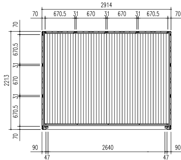
平面図 (S=1/50)
