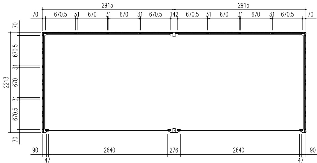
平面図 (S = 1/50)
