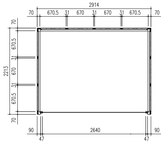
平面図 (S = 1/50)
