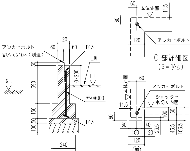
A ~ A' 断面 布基礎断面図例 (S = 1/20)
