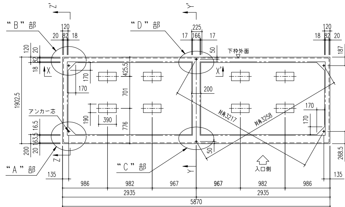
基礎伏図 (S=1/50)
