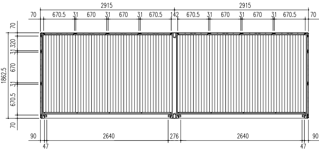
平面図 (S = 1/50)
