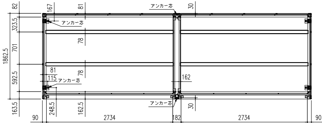
床伏図 (S = 1/50)
