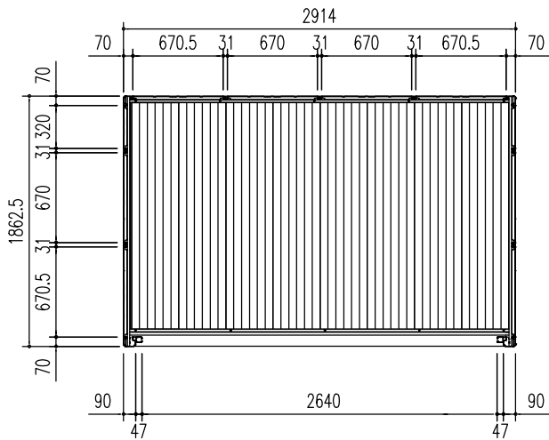
平面図 (S=1/50)
