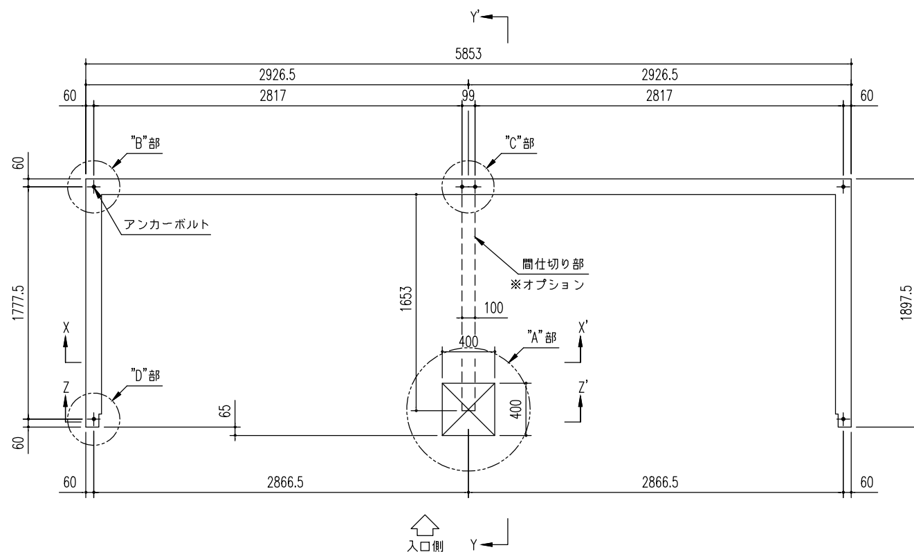
基礎伏図 (S=1/40)
