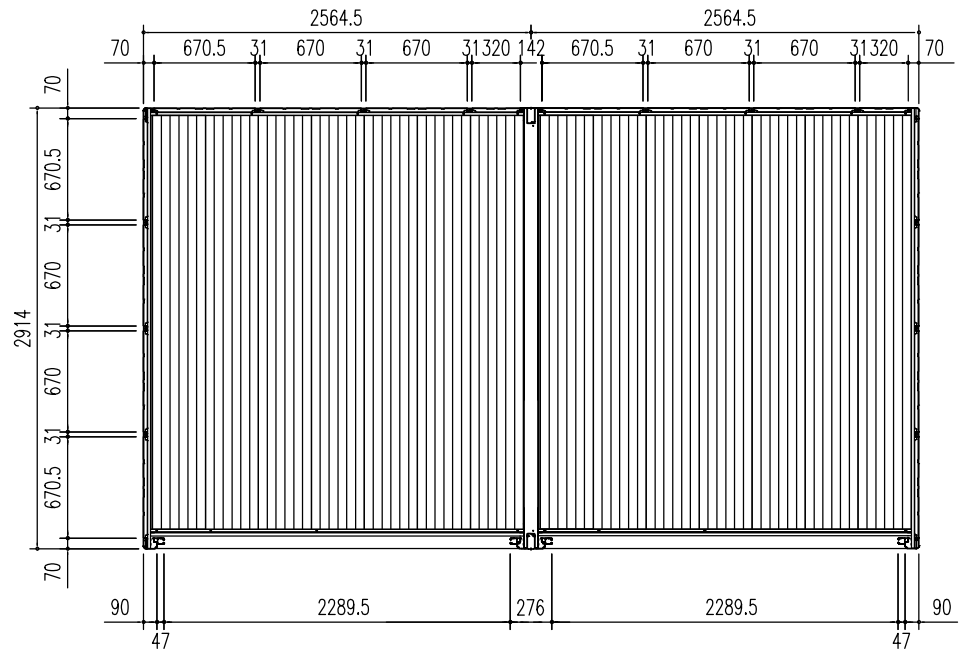
平面図 (S = 1/50)
