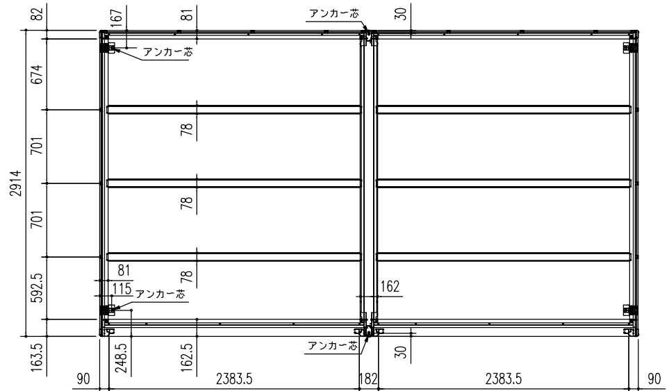
床伏図 (S = 1/50)
