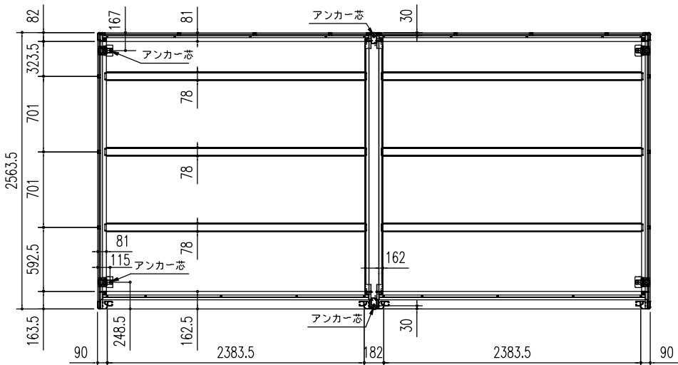
床伏図 (S = 1/50)
