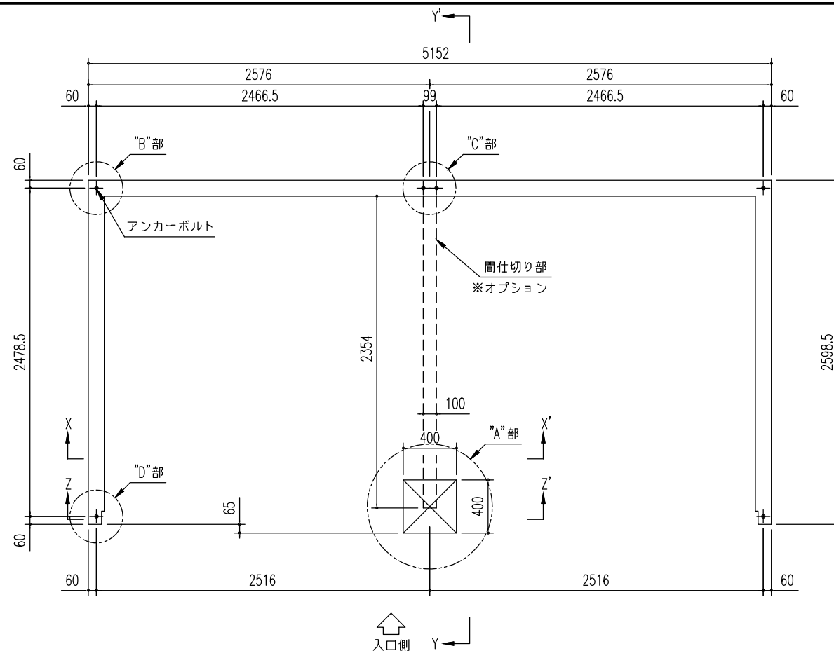
基礎伏図 (S=1/40)
