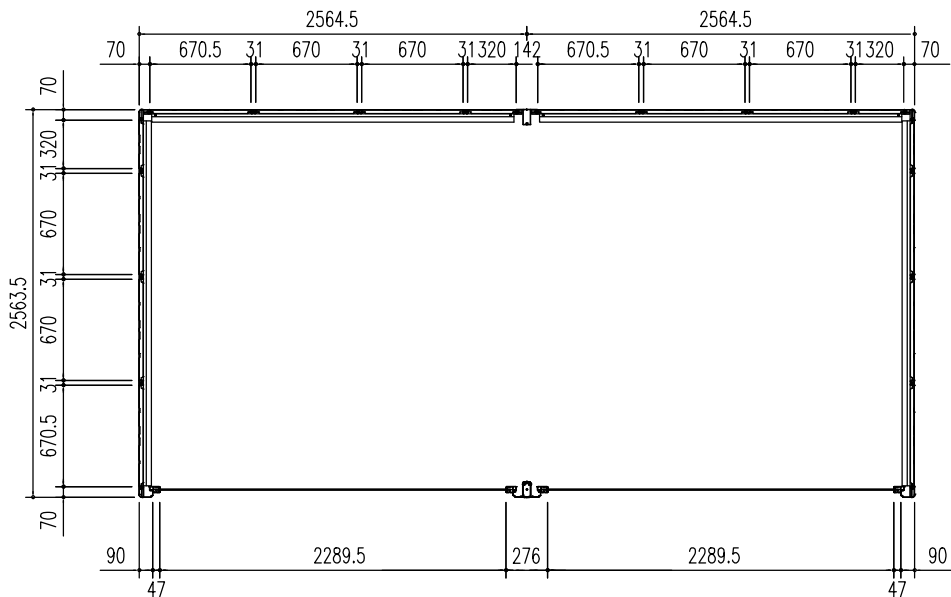
平面図 (S = 1/50)
