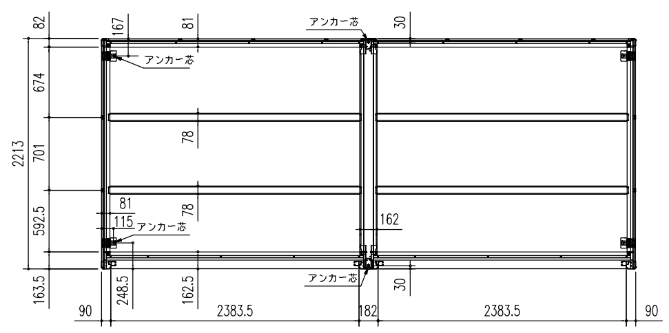
床伏図 (s = 1/50)
