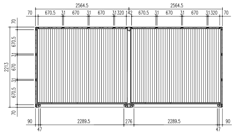
平面図 (s = 1/50)
