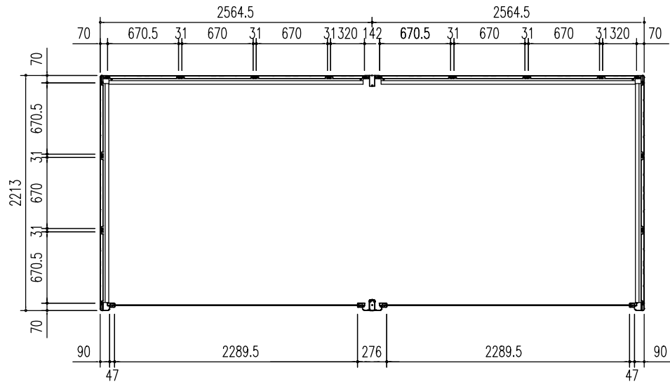
平面図 (S = 1/50)
