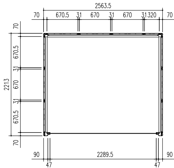
平面図 (S=1/50)
