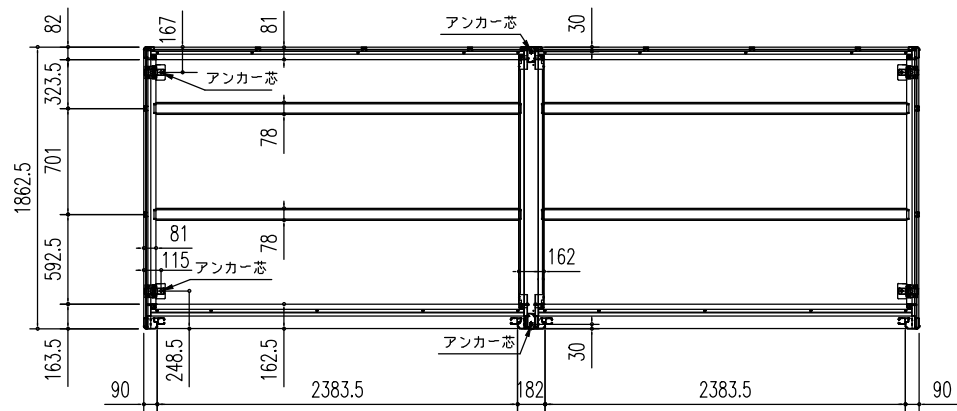
床伏図 (S = 1/50)
