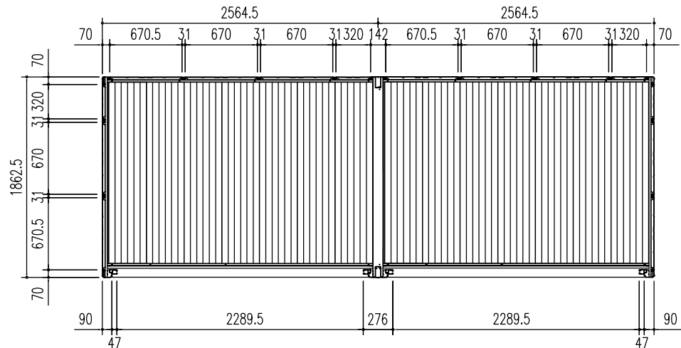
平面図 (S = 1/50)
