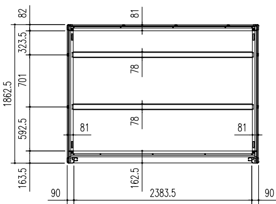
床伏図 (S=1/50)
