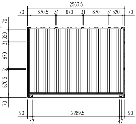
平面図 (S=1/50)
