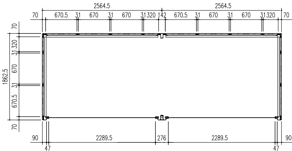
平面図 (S=1/50)
