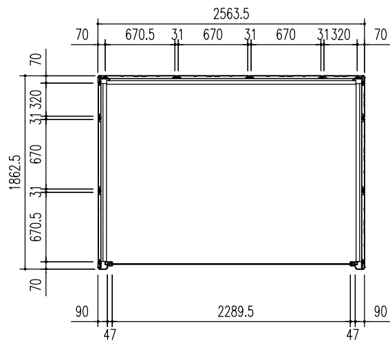
平面図 (S=1/50)
