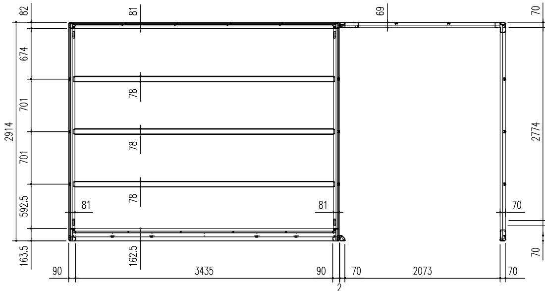
床伏図 (S = 1/50)
