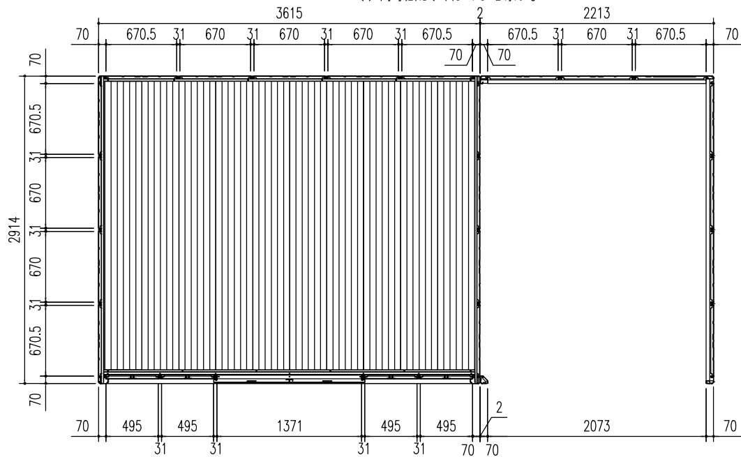
平面図 (S = 1/50)
