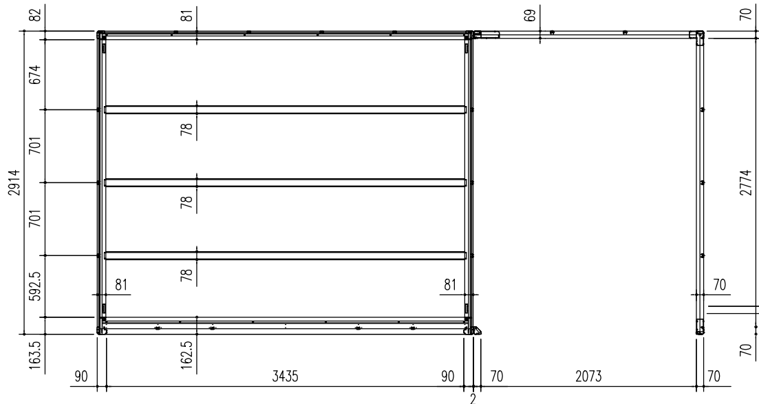
床伏図 (S = 1/50)
