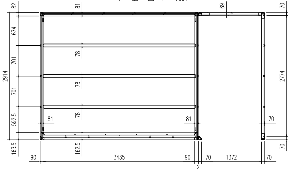
床伏図 (S = 1/50)
