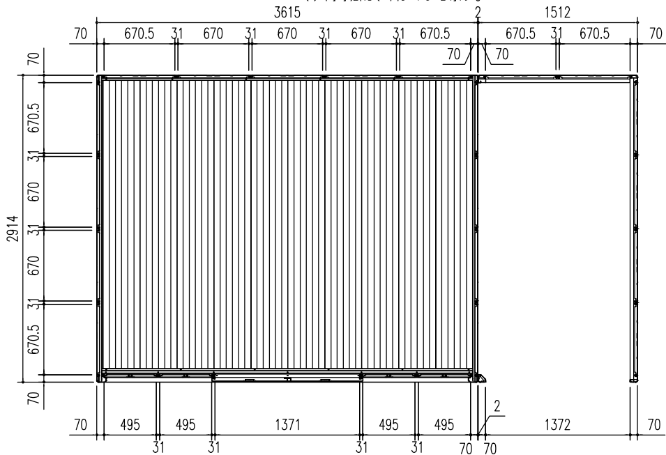
平面図 (S = 1/50)
