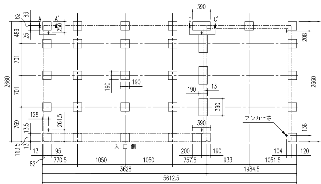
ブロック基礎伏図 (S = 1/50) (内アンカー用) ※内アンカーセット (オプション) 別途必要 ※オープン部には付属のアンカープレート (L) を使用
