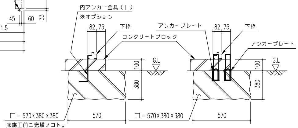
C ~ C' 断面 (内アンカー用) D ~ D' 断面 (外アンカー用) ブロック基礎断面図例 (S = 1/20)
