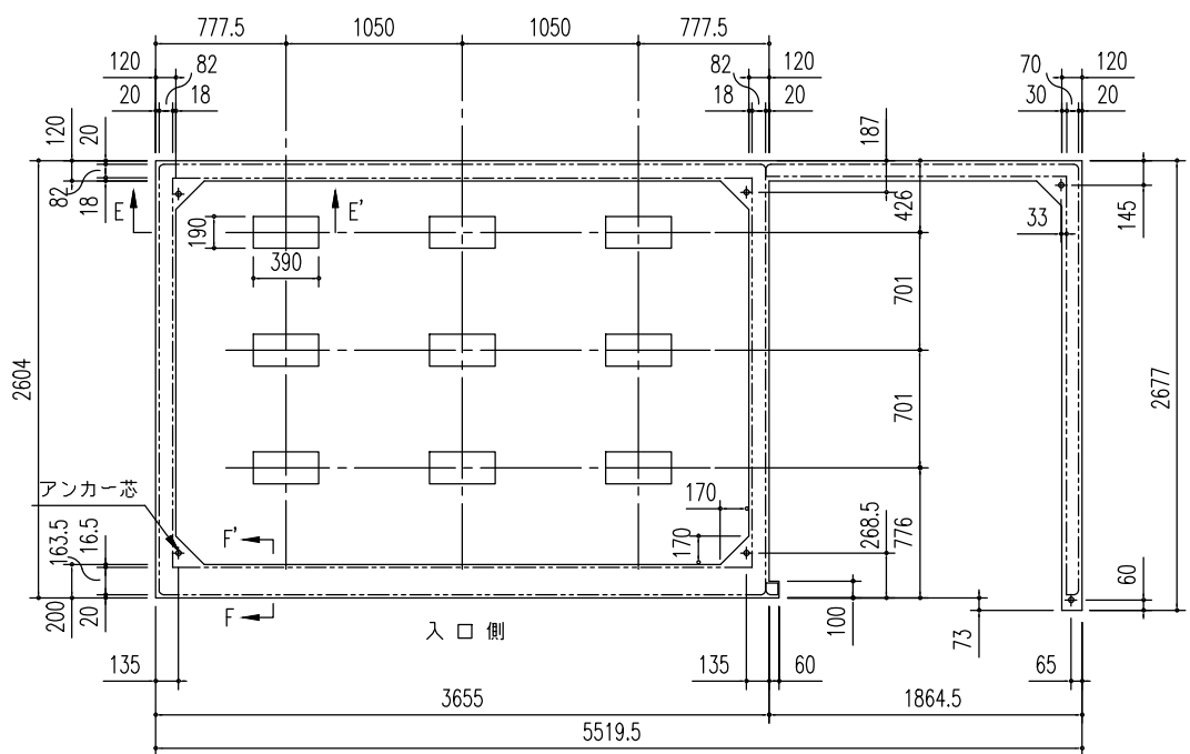
布基礎伏図 (S = 1/50) ※内アンカーセット (オプション) 別途必要 ※オープン部には付属のアンカープレート (L) を使用
