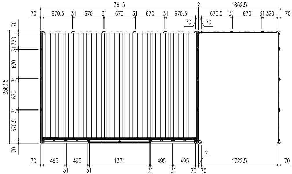
平面図 (S = 1/50)
