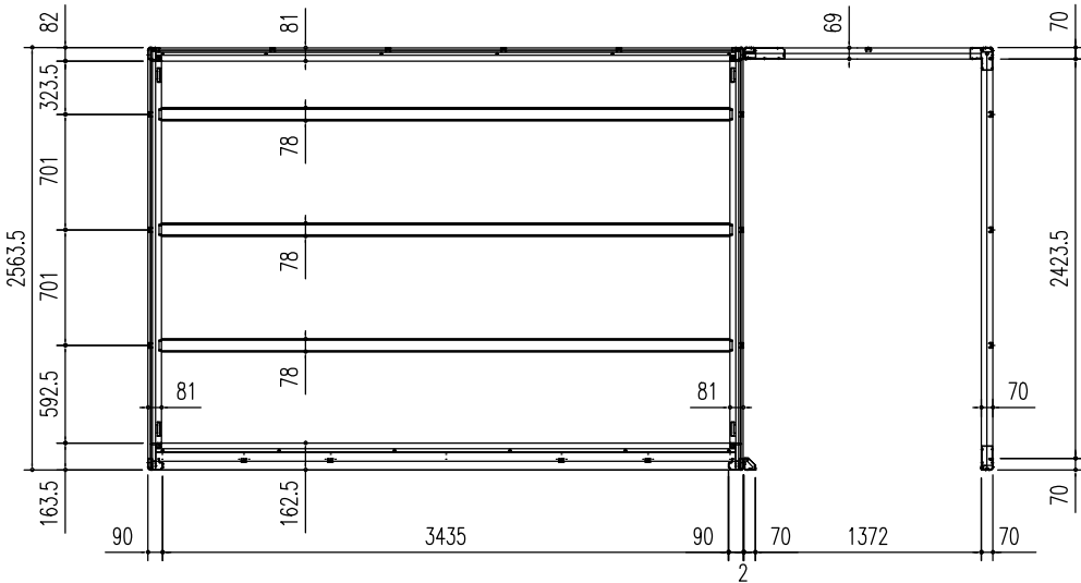
床伏図 (S = 1/50)
