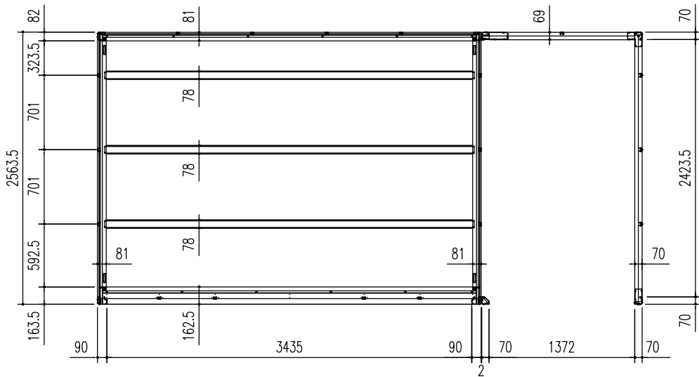
床伏図 (S = 1/50)
