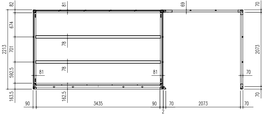
床伏図 (S = 1/50)
