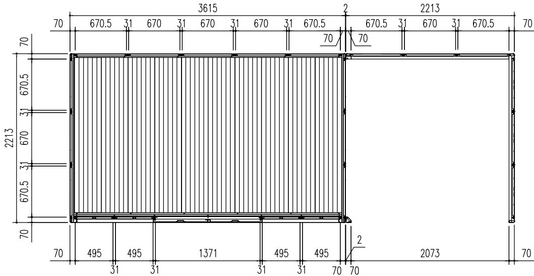
平面図 (S = 1/50)
