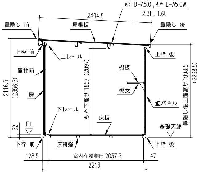
〔物置部〕矩計図 (S = 1/50)
