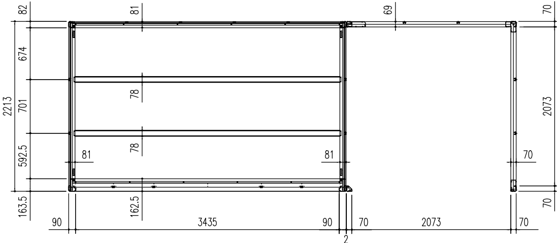
床伏図 (S = 1/50)
