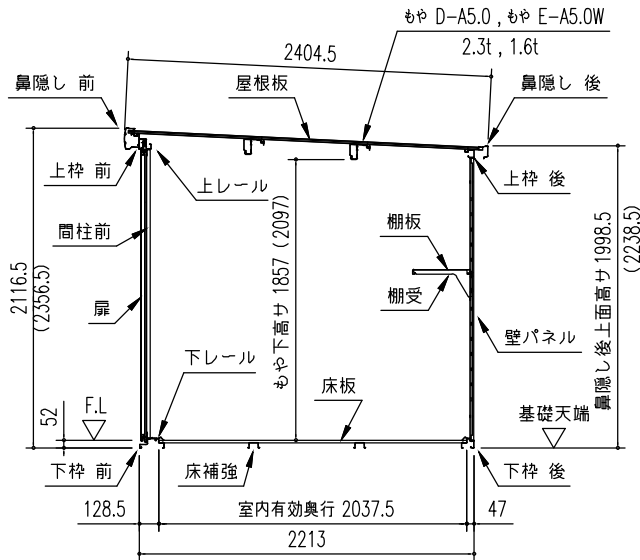
[物置部] 矩計図 (S = 1/50) ※ ( ) 内寸法は、Hタイプを示す。
