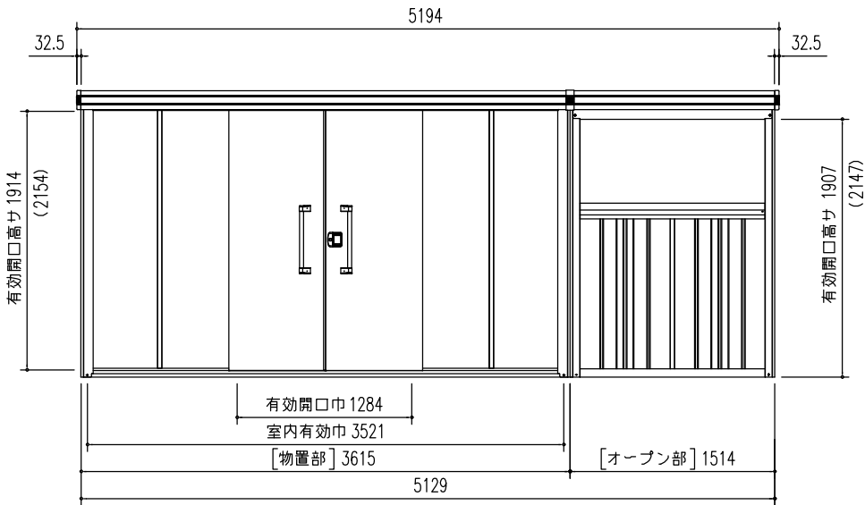
正面立面図 (S = 1/50) ※ ( ) 内寸法は、Hタイプを示す。
