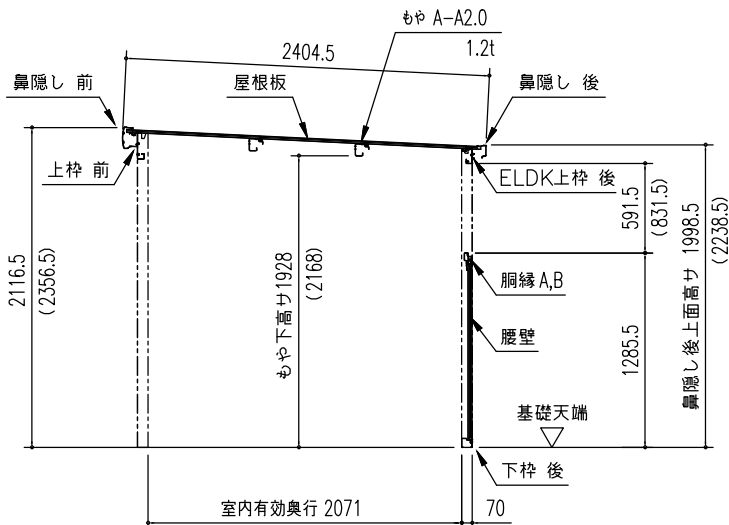
[オープン部] 矩計図 (S = 1/50) ※ ( ) 内寸法は、Hタイプを示す。
