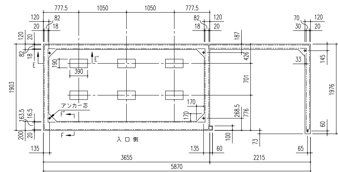
布基礎伏図 (S=1/50)
