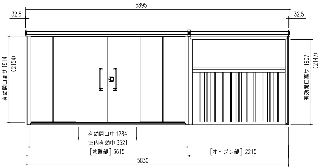
正面立面図 (S = 1/50) ※ ( ) 内寸法は、Hタイプを示す。
