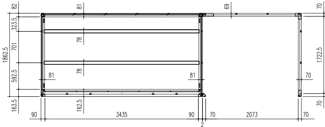
床伏図 (S = 1/50)
