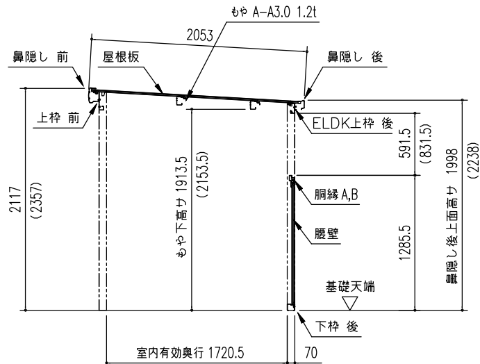
「オープン部」矩計図 (S = 1/50) ※ ( ) 内寸法は、Hタイプを示す。
