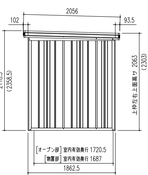
側面立面図 (S = 1/50) ※ ( ) 内寸法は、Hタイプを示す。
