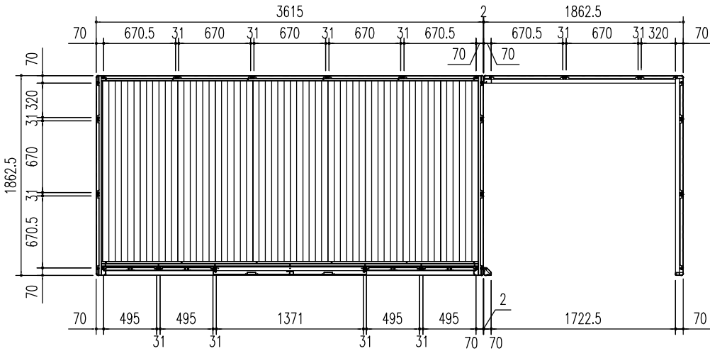
平面図 (S = 1/50)
