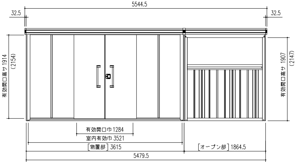
正面立面図 (S = 1/50) ※ ( ) 内寸法は、Hタイプを示す。
