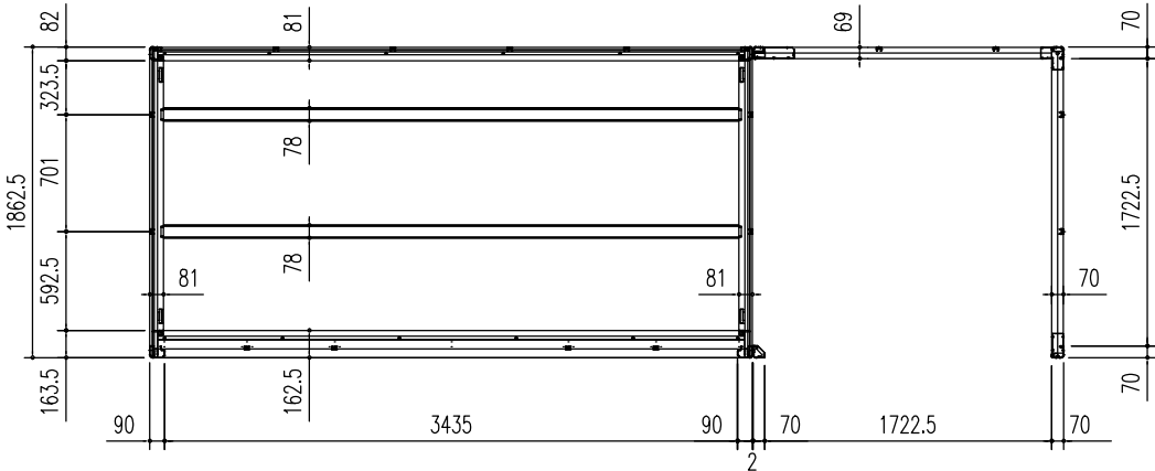
床伏図 (S = 1/50)
