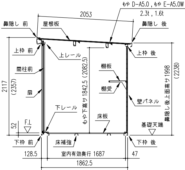
〔物置部〕矩計図 (S = 1/50) ※ ( ) 内寸法は、Hタイプを示す。
