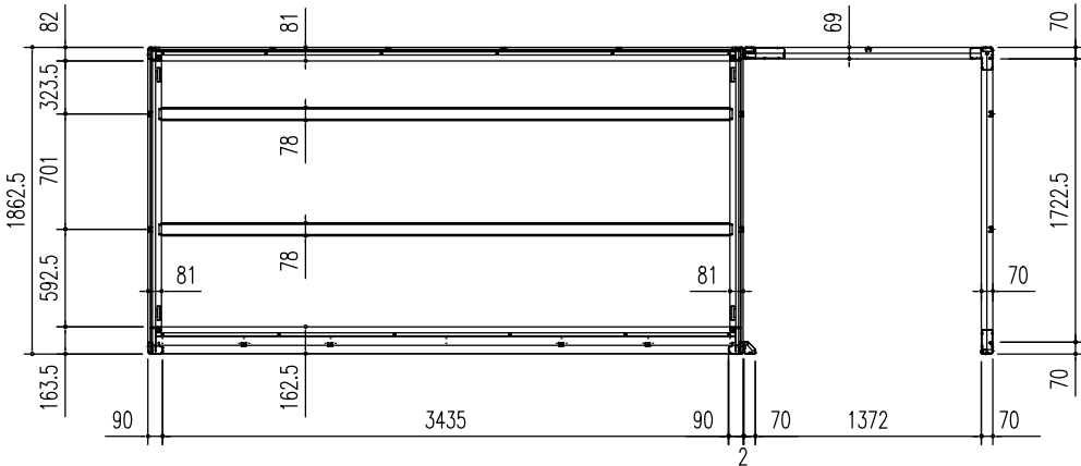
床伏図 (S=1/50)
