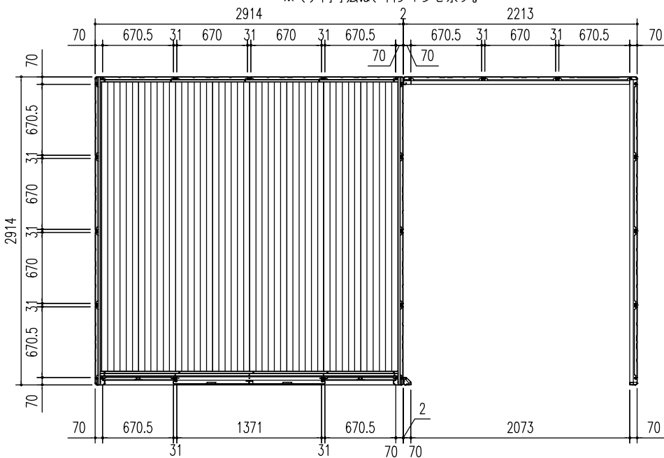
平面図 (S = 1/50)
