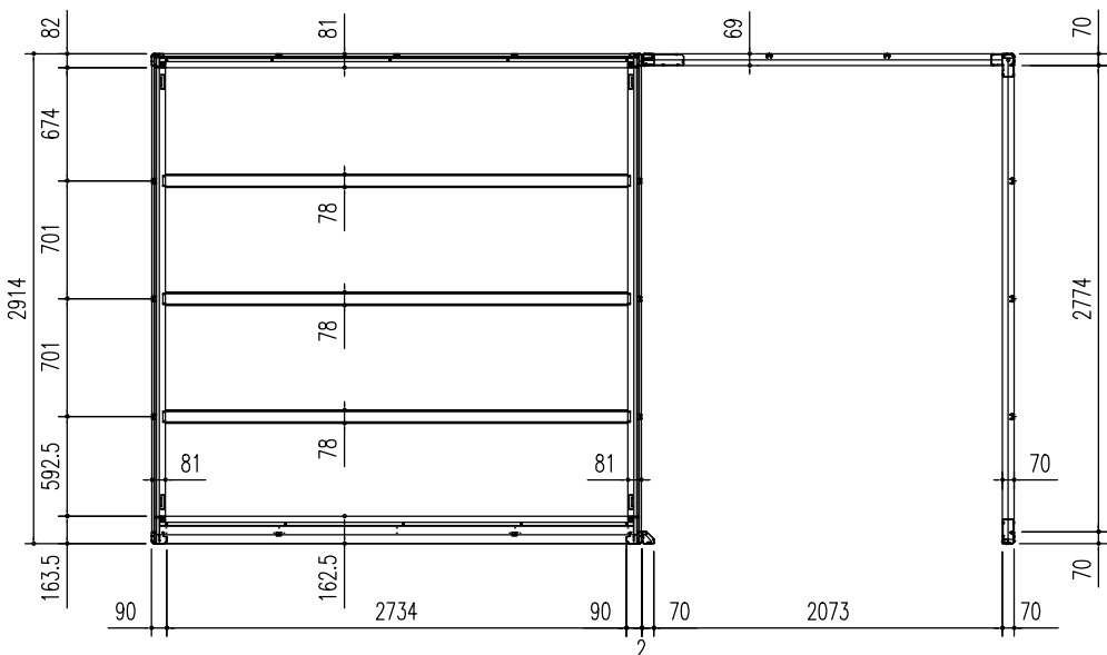
床伏図 (S = 1/50)
