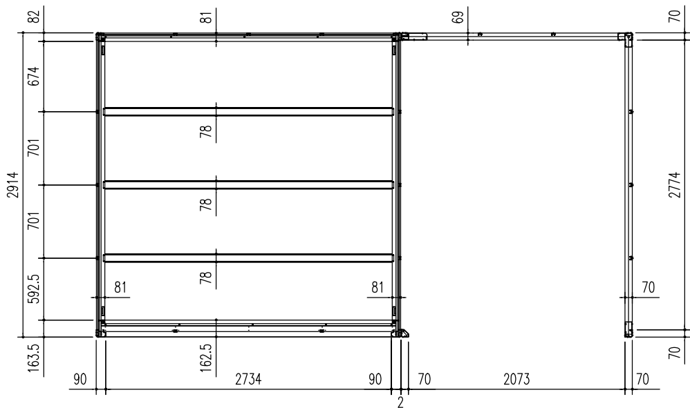
床伏図 (S = 1/50)
