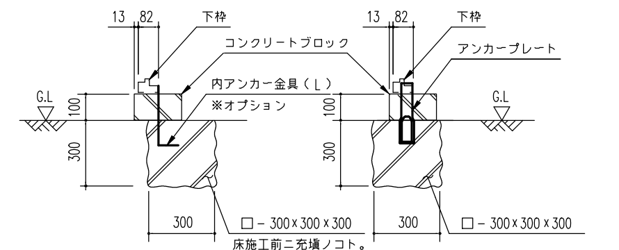
A ~ A' 断面 (内アンカー用) B ~ B' 断面 (外アンカー用)
