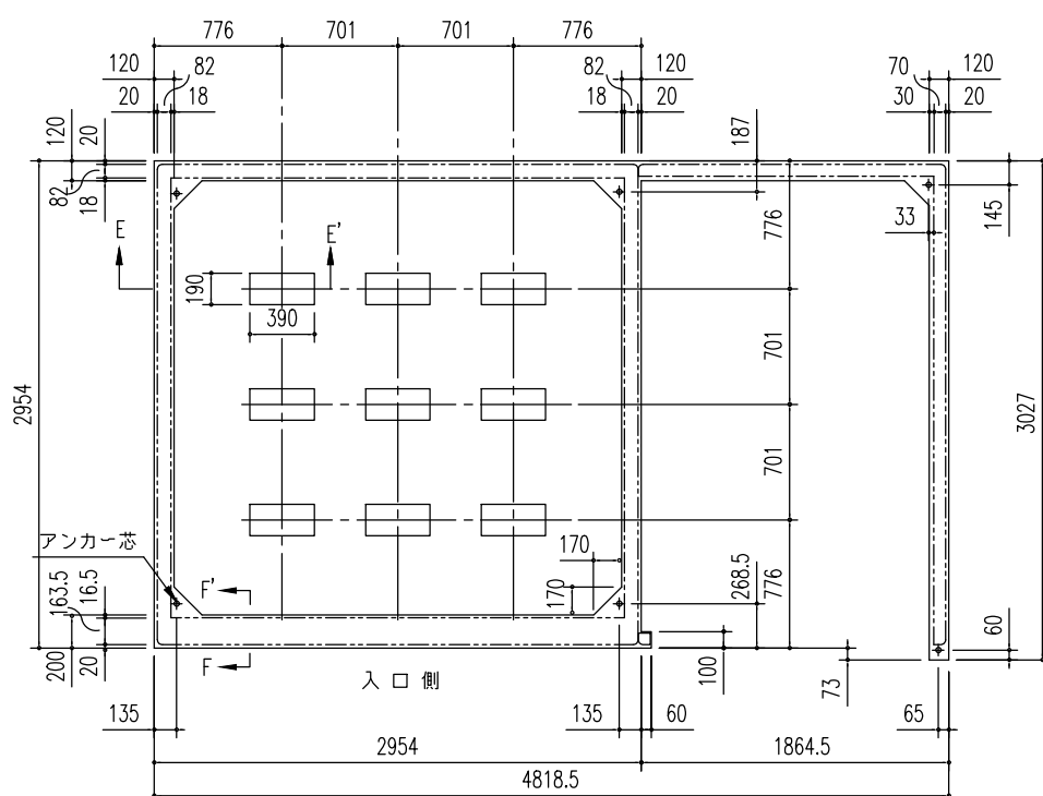
布基礎伏図 (S=1/50)
