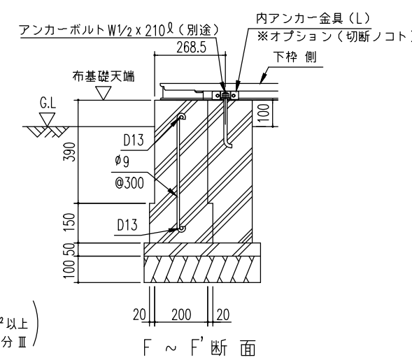
F ~ F' 断面
