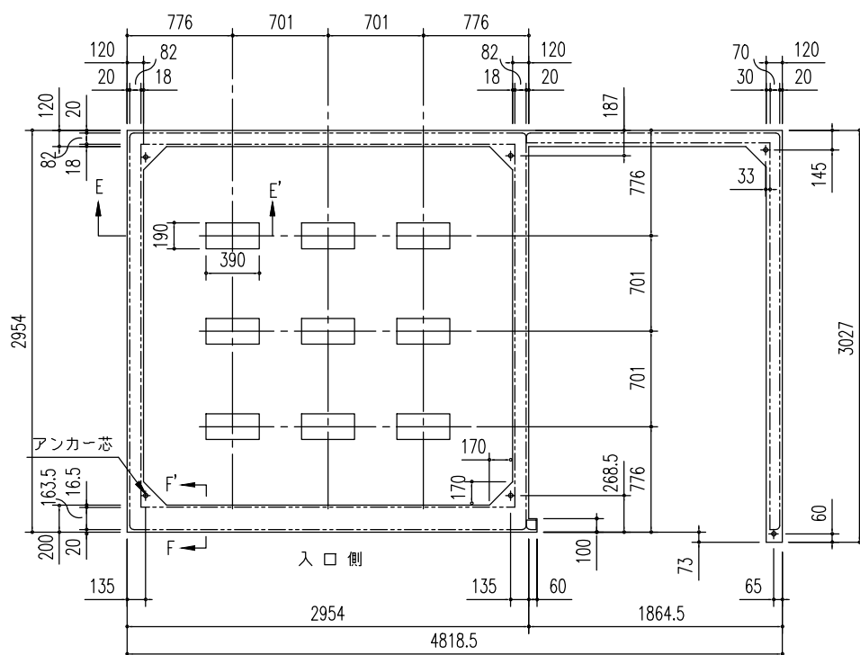
布基礎伏図 (S=1/50) ※内アンカーセット (オプション) 別途必要 ※オープン部には付属のアンカープレート (L) を使用
