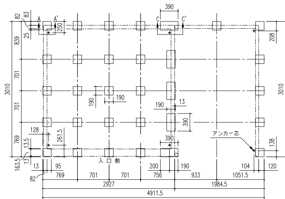
ブロック基礎伏図 (S=1/50) (内アンカー用) ※内アンカーセット (オプション) 別途必要 ※オープン部には付属のアンカープレート (L) を使用
