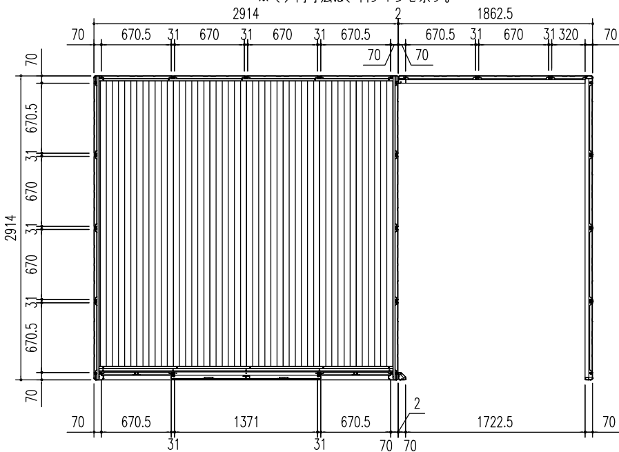
平面図 (S=1/50)
