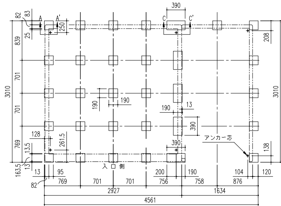
ブロック基礎伏図 (S=1/50) (内アンカー用) ※内アンカーセット (オプション) 別途必要 ※オープン部には付属のアンカープレート (L) を使用
