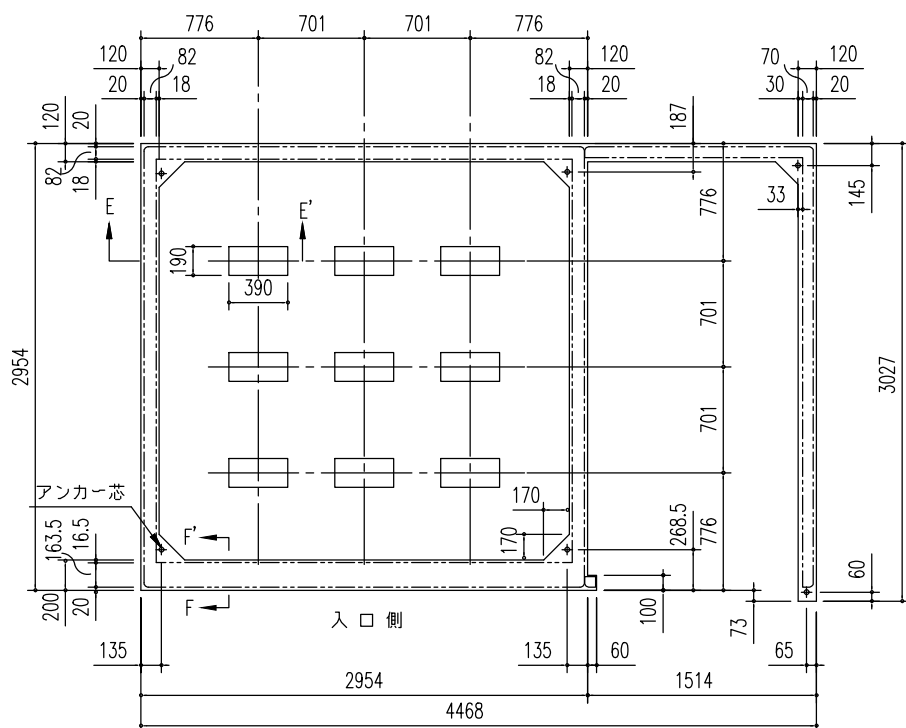
布基礎伏図 (S=1/50) ※内アンカーセット (オプション) 別途必要 ※オープン部には付属のアンカープレート (L) を使用
