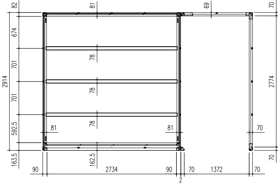
床伏図 (S=1/50)
