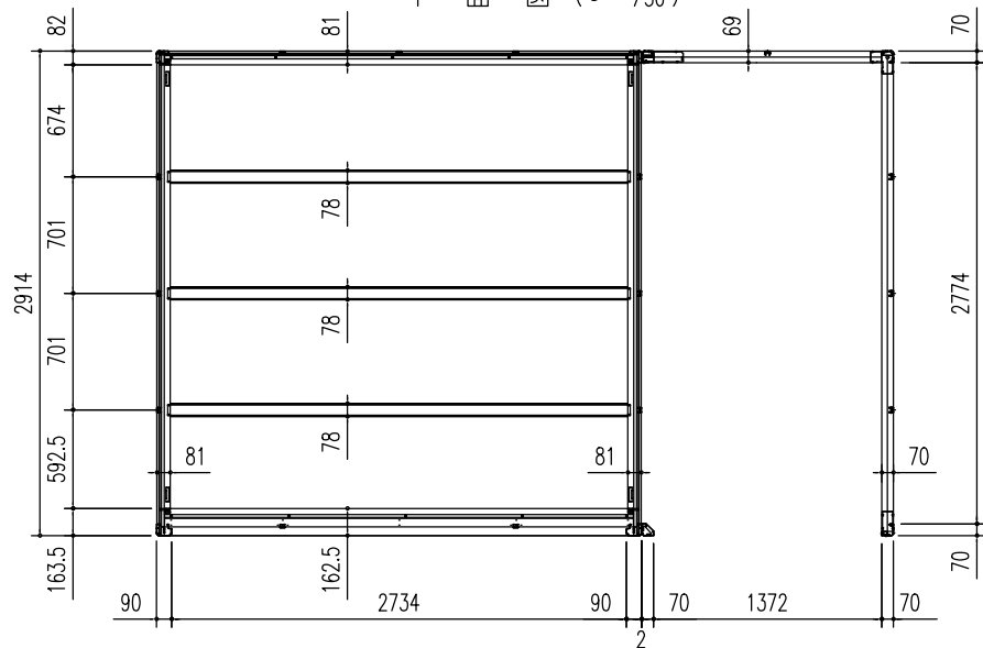
床伏図 (S = 1/50)
